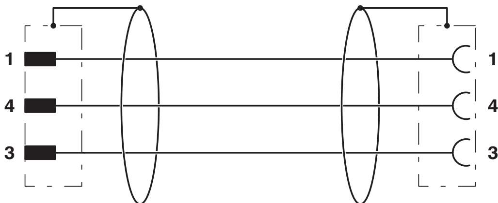
Disposition des contact des connecteurs mâles/femelles M8
