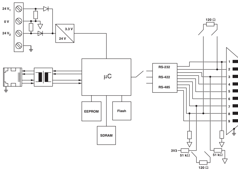
Schéma fonctionnel
