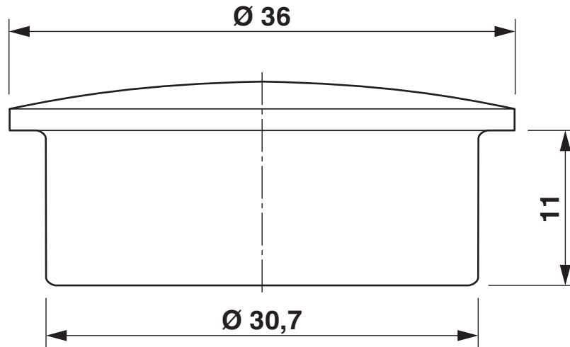
Maßzeichnung
