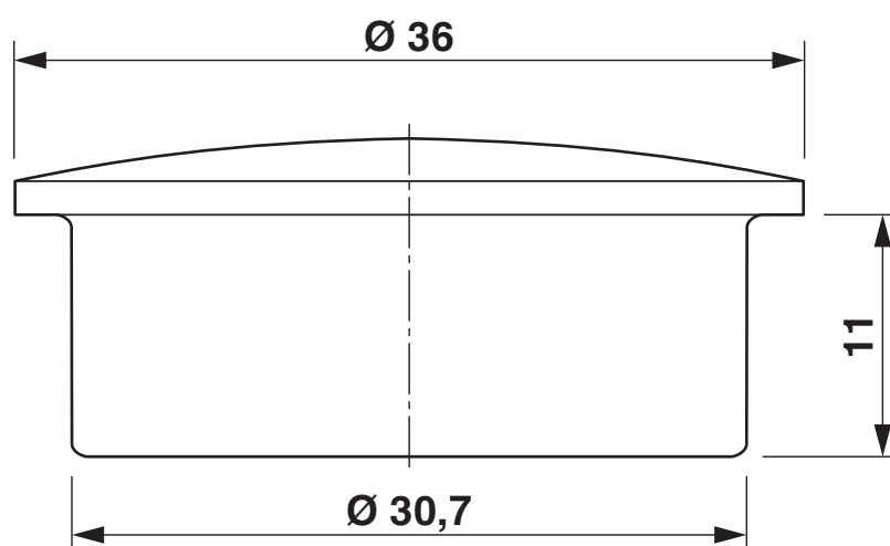
Dessin coté
