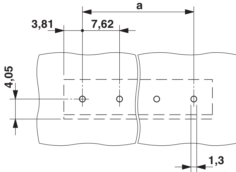
Bohrplan/Lötpadgeometrie
