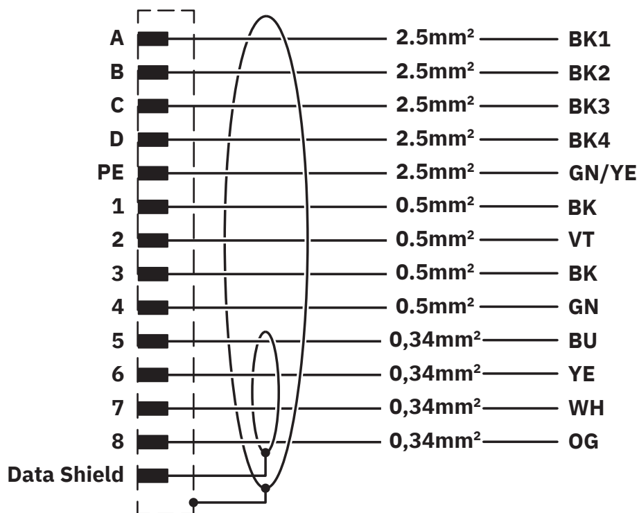
Diagrama eléctrico
