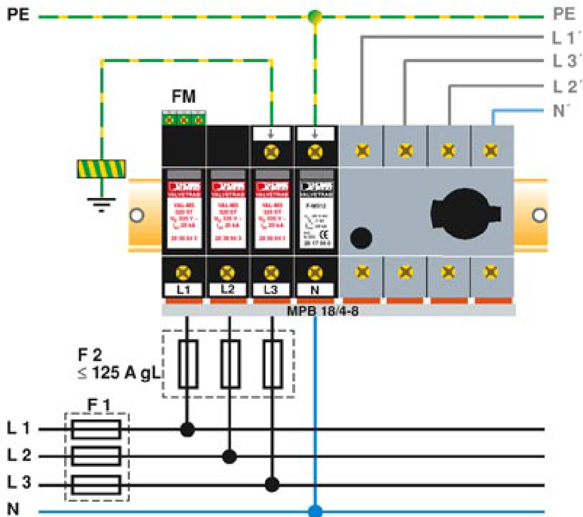
Applikationszeichnung
