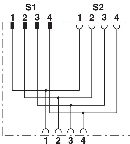
Schaltplan
