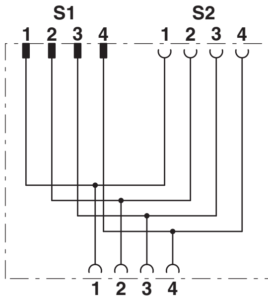
Diagrama eléctrico
