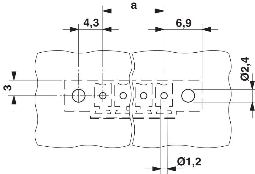
Bohrplan/Lötpadgeometrie
