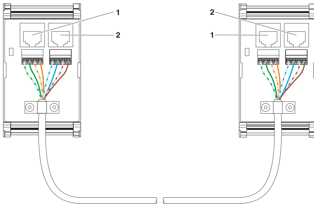
Anschlusszeichnung
