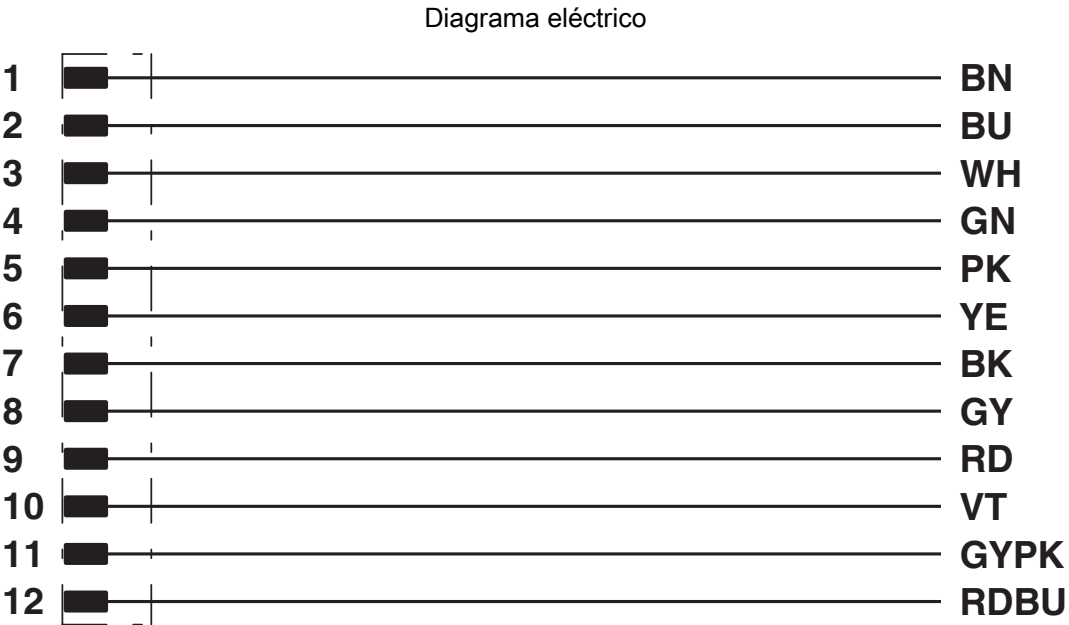
Ocupación de contactos del conector macho M12
