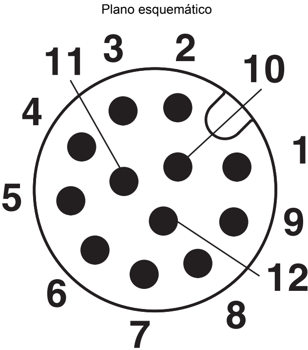
Esquema de polos del conector macho M12, 12 polos, vista de la cara de machos
