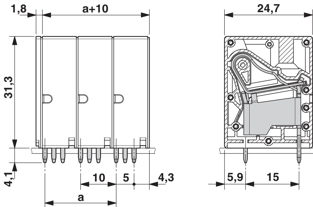
Maßzeichnung
